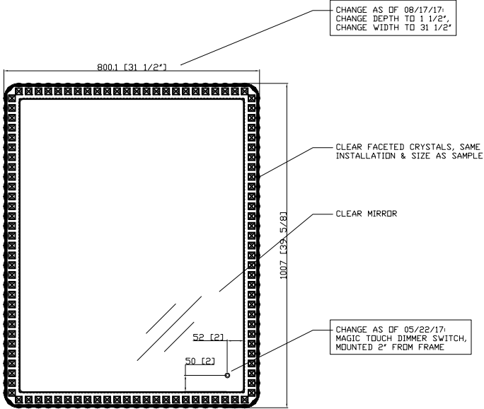
ELEVATION - TOP
