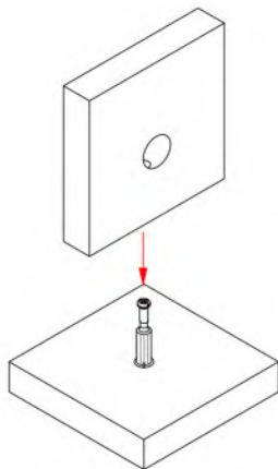
4. Die Montageplatte
