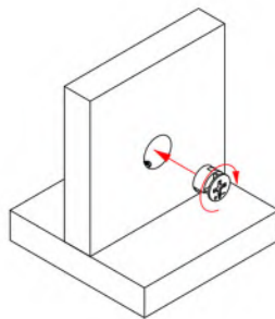
5. Den Pfeil des exzentrischen Bauteils auf die Gewindestange ausrichten
