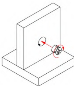
5. aligner la flèche du composant excentrique avec la tige de vis
